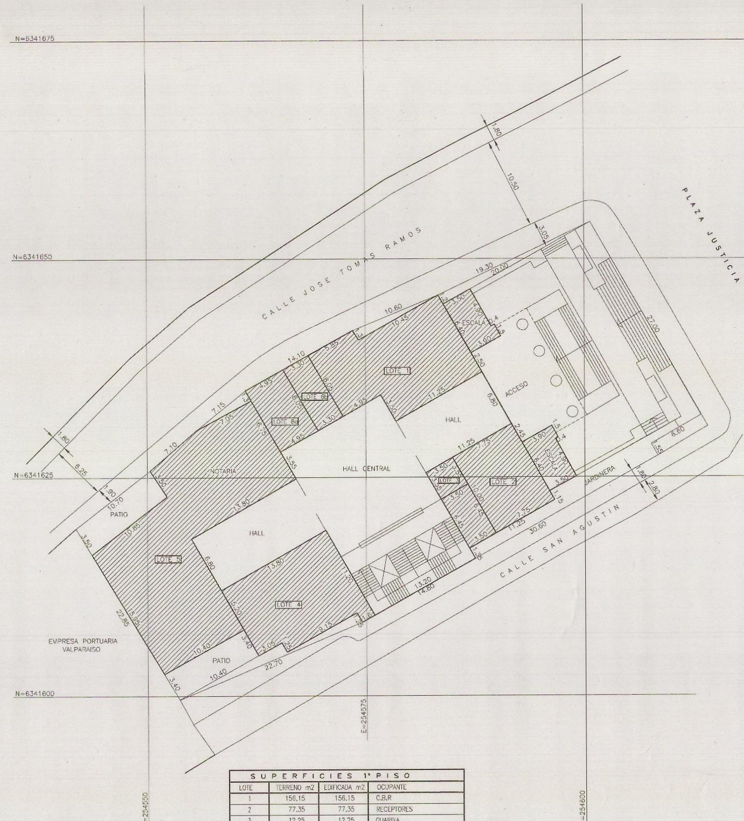
PLANTA 1° NIVEL
