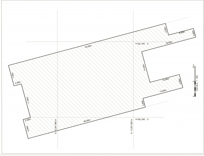
PLANTA SUBTERRANEO SUPERFICIE CONSTRUIDA : 1190,95 m 2
